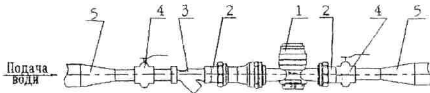
Рис. 4 Рекомендована схема встановлення лічильника води
